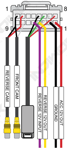
AV CABLE
