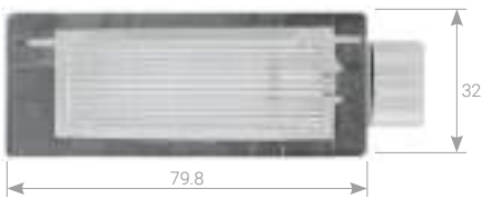
PLL-071 Luci di Targa License Plate Lights
