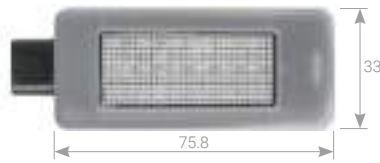
PLL-072 Luci di Targa License Plate Lights
